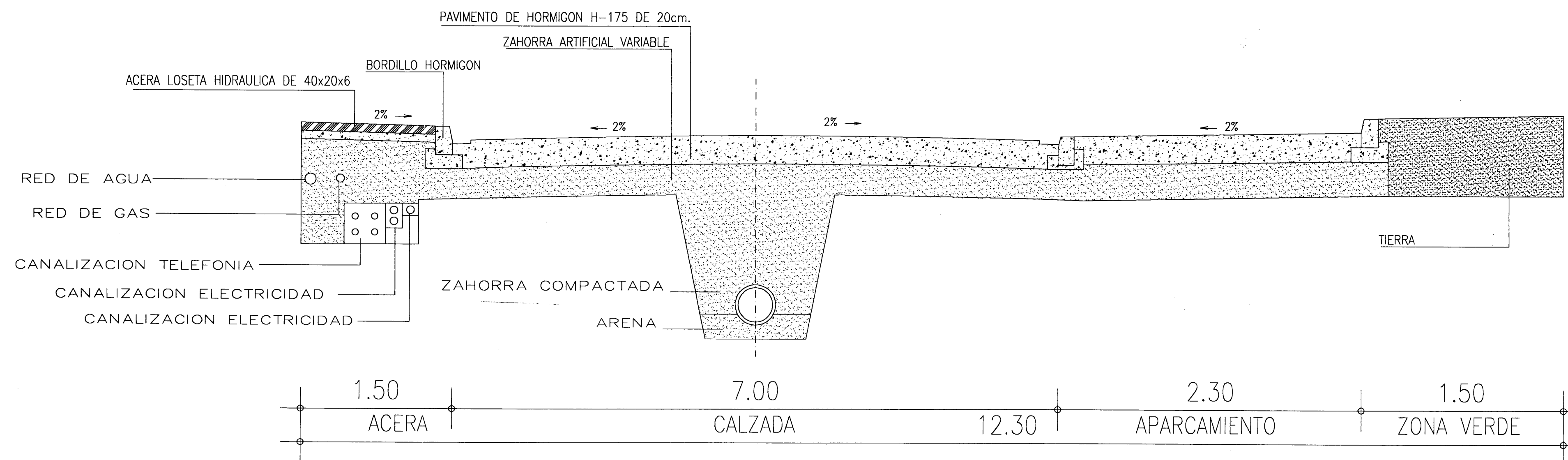
SECCION A-A
