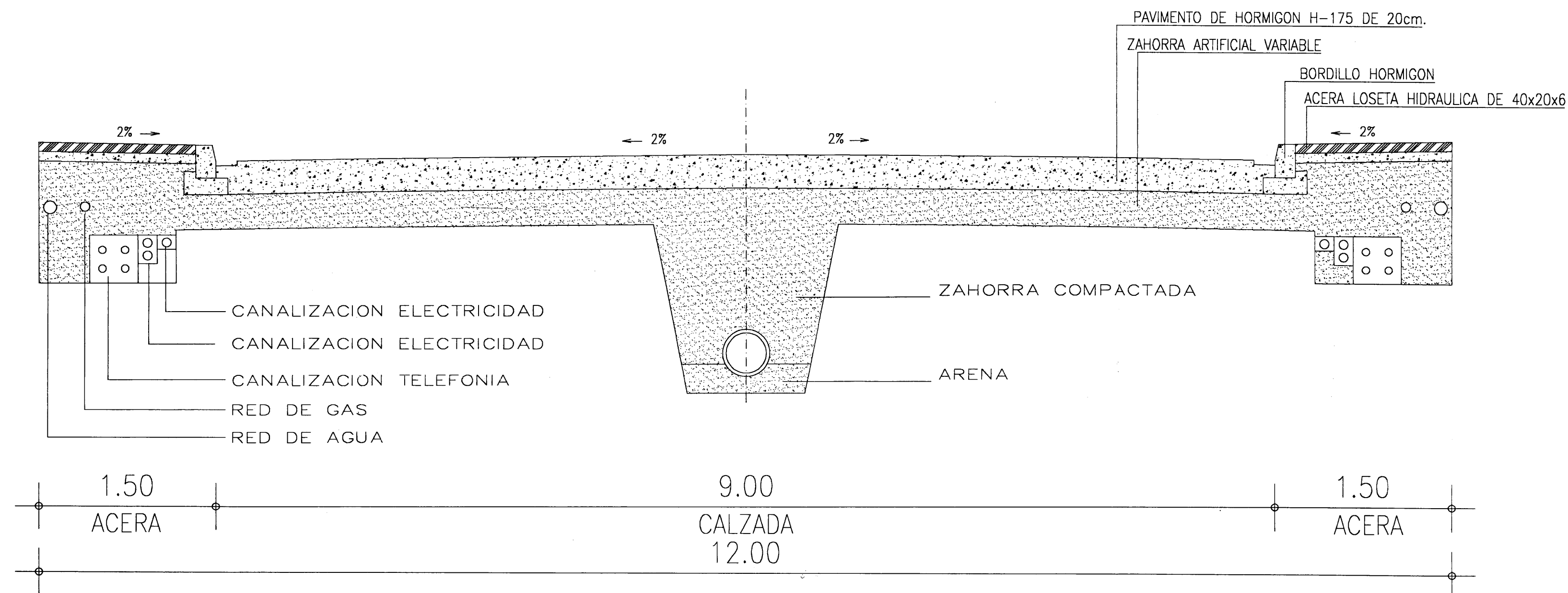
SECCION B-B, C-C
